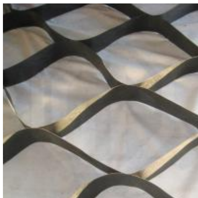
ОР-5 СНО Георешетка облегченная 5см 160x160мм толщина 1,2мм
