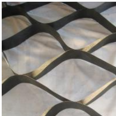
ОР-5 СН Георешетка полимерная 5см 160x160мм толщина 1,5мм
