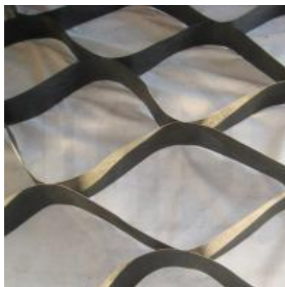
ОР-5 С Георешетка полимерная 5см 210x210мм толщина 1,5мм
