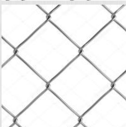
Сетка плетеная рабица оцинкованная 50x50мм d3мм
