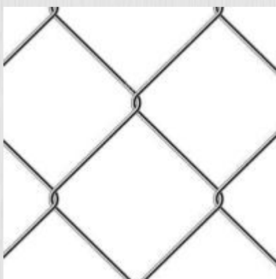
Сетка плетеная рабица оцинкованная 65x65мм d2,8мм
